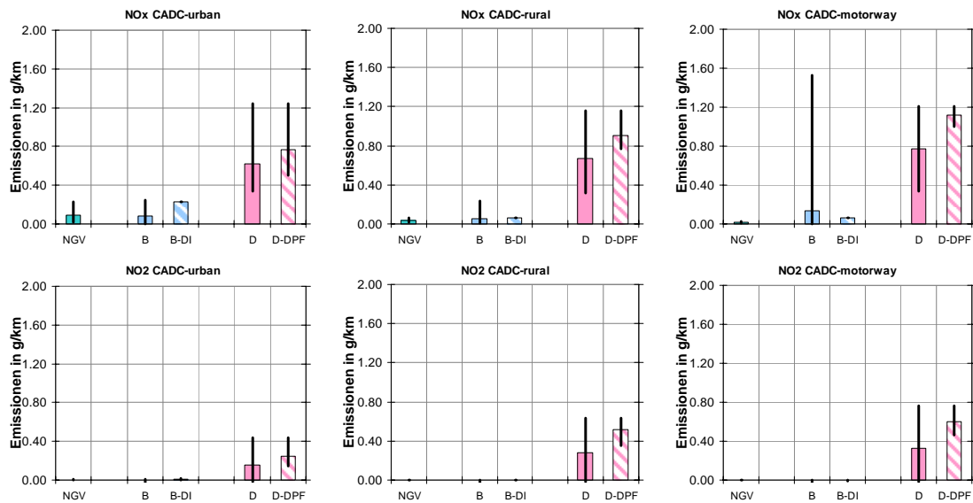
Abb. 16 Stickoxidemissionen NO x (obere Reihe) und Stickstoffdioxidemissionen NO 2 (untere Reihe) im Artemis-Fahrzyklus
