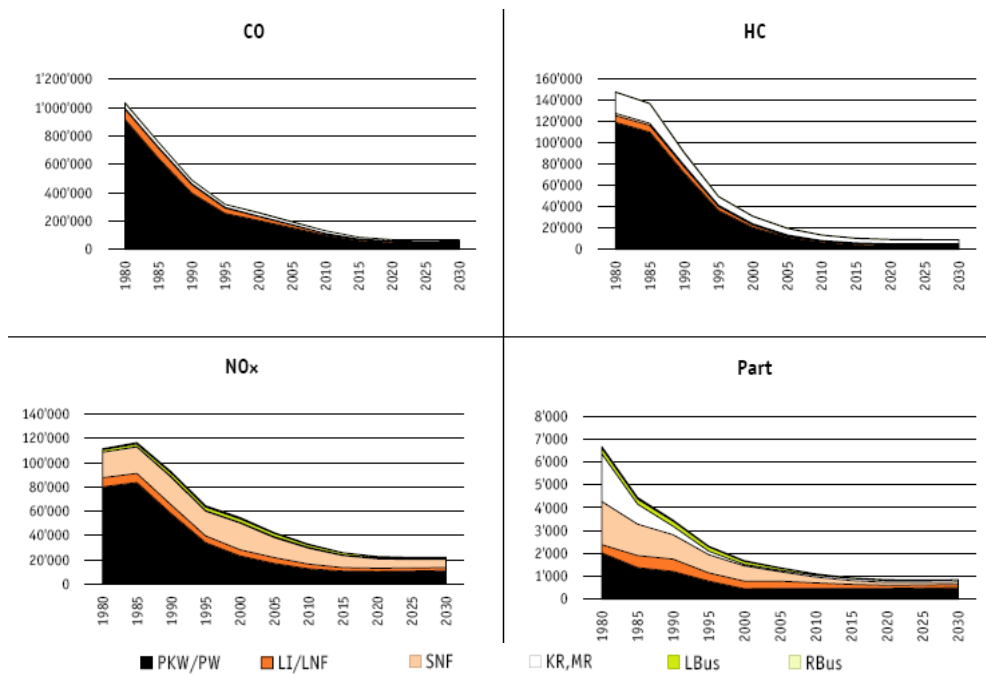
Abb. 2 Emissionsentwicklung 1980 - 2030 [T/a] nach Fahrzeugkategorie (Quelle: BAFU)
